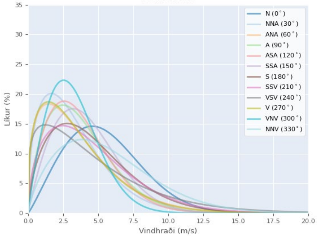
Weibull Vor
