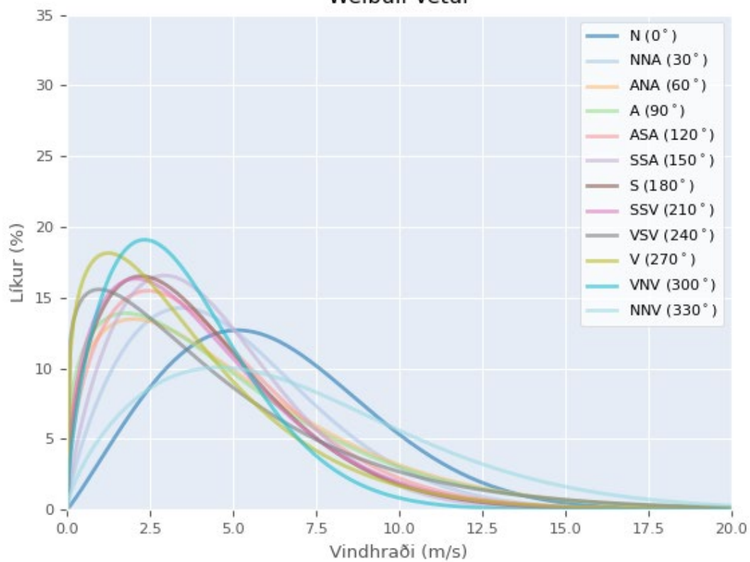
Weibull Vetur
